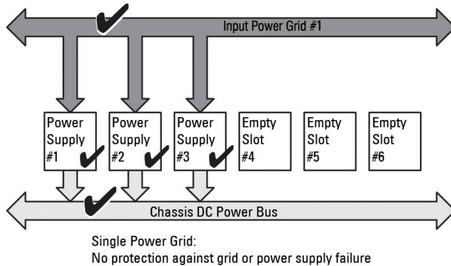
Abbildung 7. „Keine Redundanz“ bei drei Netzteilereinheiten im Gehäuse
